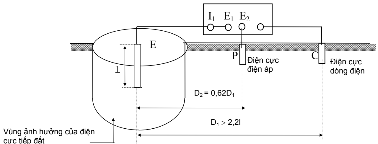
Hình A.2 - Sơ đồ đo điện trở tiếp đất của điện cực thẳng đứng
